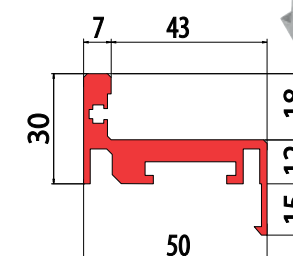
Alu dovratnik 5700 mm IG AD 5700 "Z"
