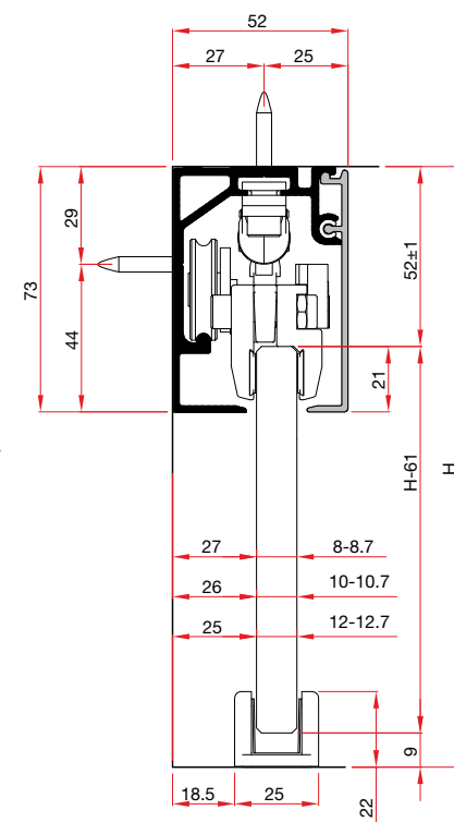
Vodilica
