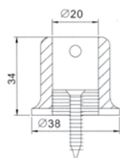
Konektor* fiksni zid-šipka
