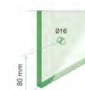
Bočni nosač za staklo 60x40
