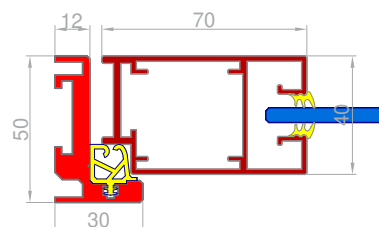
Alu dovratnik IG AD 5700 + ALU profil IG AO
