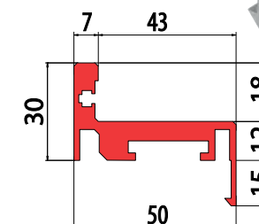
Alu dovratnik 5700 mm IG AD 5700 "Z"
