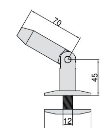
Konektor za nadstrešnicu staklo-šipka SA 8300E-2 INOX 304 / INOX 316
