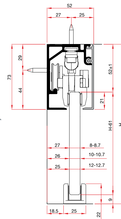
Vodilica
