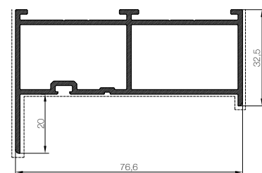
Bočni profil 3 krila
