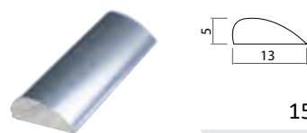
Prag 1500 mm, aluminij TA PS-59AL
