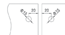
Spojnica kutna 90° inox SAT / inox POL debljina stakla 8/10/12 mm
