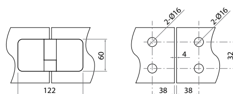
Podizna spojnica staklo-staklo debljina stakla 8/10 mm lijeva / desna
