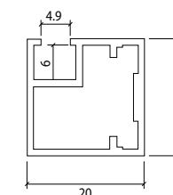
Alu profil za staklo debljina stakla 4 mm
