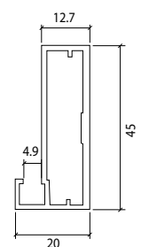
Alu profil za staklo debljina stakla 4 mm
