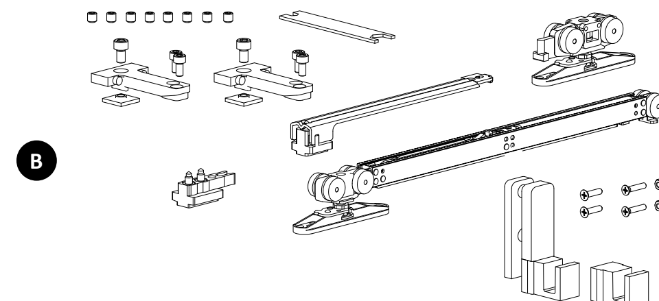
set za srednje krilo V 0342.5
