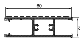
Nosáč stakla
