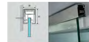
Kotač gornje vodilice
