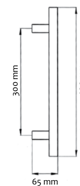
Rukohvat dužina 400 mm promjer Ø18 mm priprema stakla Ø12 mm u paru LA 1299
