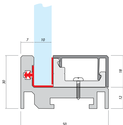
Brtva m' IG AD KLIK BRTVA I crna / siva
