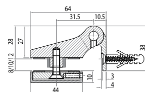
Spojnica ALU/staklo* AN debljina stakla 8/10 mm nosivost 30 kg po spojnici
