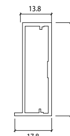
Alu profil za staklo debljina stakla 4 mm
