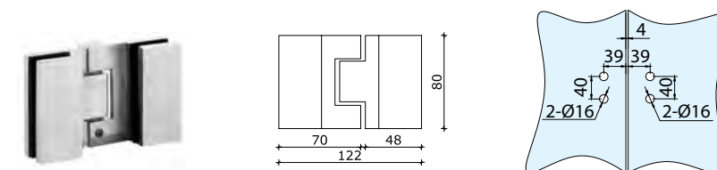
Spojnica staklo/staklo
