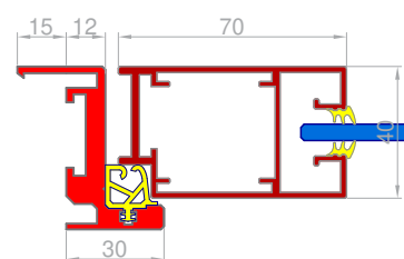
Alu dovratnik IG AD 5700 "Z" + ALU profil IG AO
