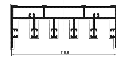
Gornji profil 5 krila
