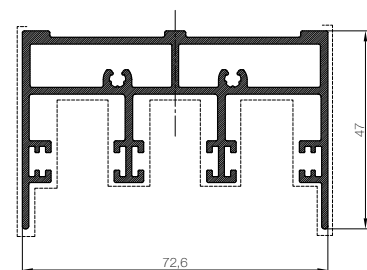
Gornji profil 3 krila
