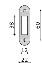
Prihvatnik brave aluminij / modro cinčano / crno
