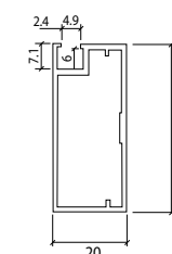
Alu profil za staklo debljina stakla 4 mm
