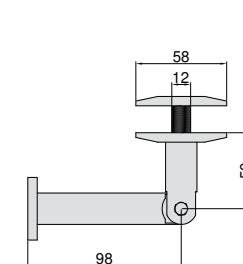
Konektor za nadstrešnicu zid-staklo SA 8300E-1 INOX 304 / INOX 316
