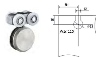
Nosač stakla
