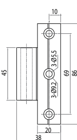
Spojnica ALU/staklo* AN debljina stakla 8/10 mm nosivost 30 kg po spojnici
