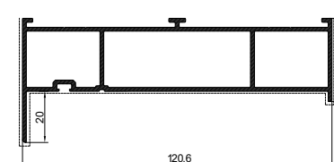
Bočni profil 5 krila
