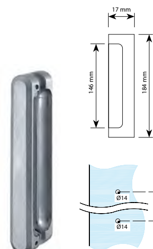
Ručica za klizna vrata razmak 161 mm priprema stakla Ø14 mm u paru
