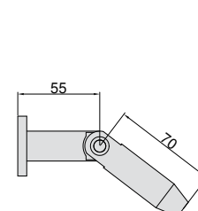
Konektor za nadstrešnicu zid-šipka SA 8300E-3 INOX 304 / INOX 316
