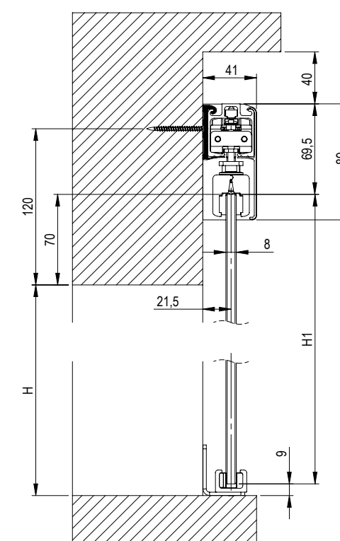
Opcija Stanlux SLX set drveno krilo
